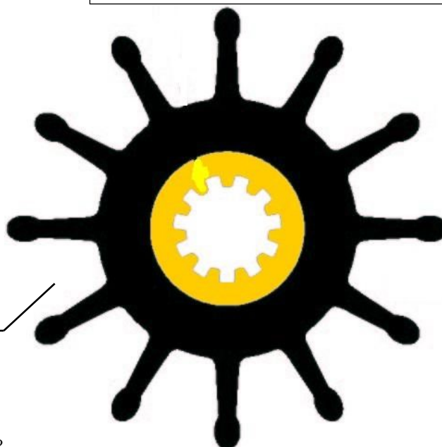
Cod. 4568: De 65 - H 50.8 - Di 16, Neoprene, Ins. 2 Cod. 4813: De 65 - H 50.8 - Di 16, Neoprene, Ins. 2
