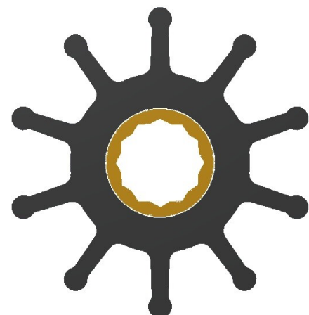
Cod. 6184: De 57 - H 50.8 - Di 16, Neoprene, Ins. 4 Cod. 6670: De 57 - H 50.8 - Di 16, Neoprene, Ins. 8
