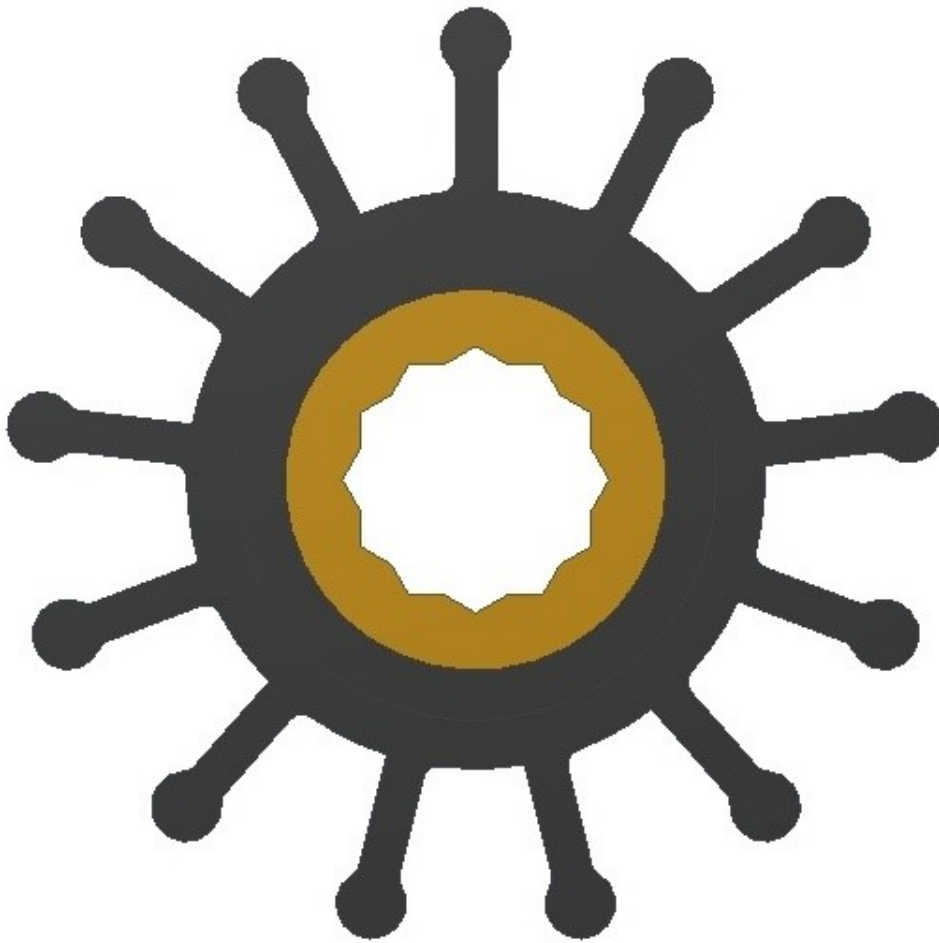
Cod. 5897: De 126.5 - H 126.8 - Di 36, Neoprene, Ins. 4
