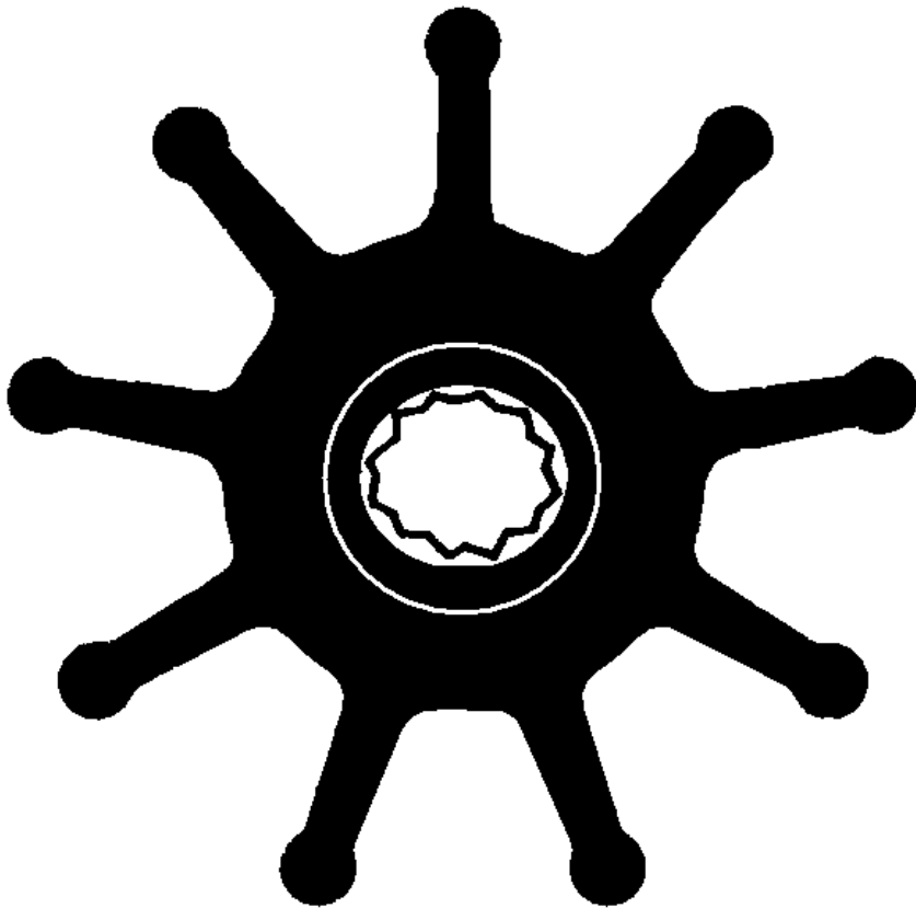
Cod. 5293: De 117 - H 130 - Di 25.4, Neoprene, Ins. 4 Cod. 4738: De 118 - H 88.5 - Di 25.4, Neoprene, Ins. 4 Cod. 4823: De 118 - H 88.5 - Di 25.4, Neoprene, Ins. 8
