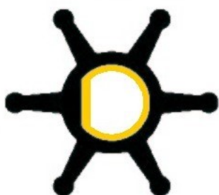
Cod. 4807: De 40 - H 19 - Di 12.1, Neoprene, Ins. 5
