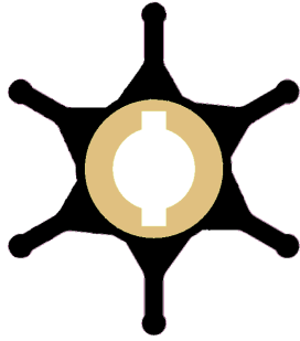
Cod. 5272: De 40 - H 14 - Di 10, Neoprene, Ins. 7
