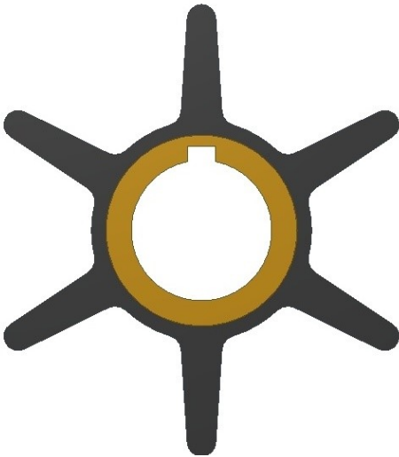
Cod. 6053: De 67.45 - H 35.1 - Di 20.1, Neoprene, Ins. 3
