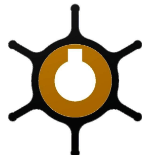
Cod. 5356: De 36 - H 14.5 - Di 9.7, Neoprene, Ins. 3
