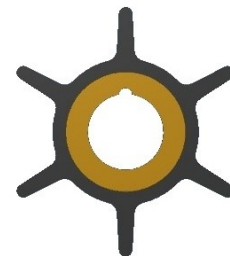
Cod. 6048: De 33.6 - H 14.4 - Di 10.3, Neoprene, Ins. 6
