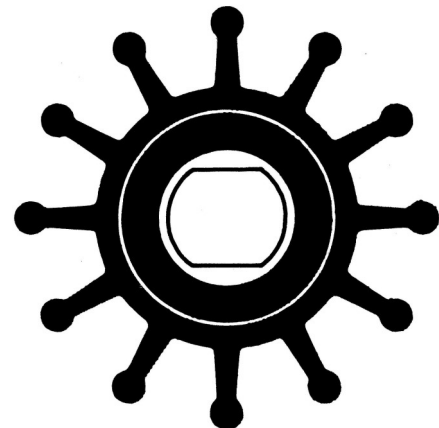
Cod. 3392: De 57 - H 31.7 - Di 16, Neoprene, Ins. 3
