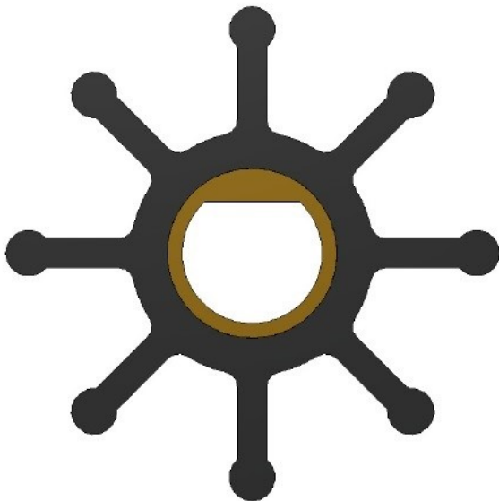
Cod. 3386: De 65 - H 50.8 - Di 19, Neoprene, Ins. 5
