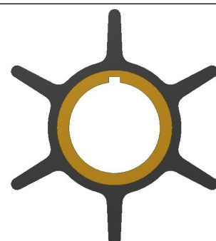
Cod. 6051: De 44.1 - H 20.25 - Di 17.1, Neoprene, Ins. 3
