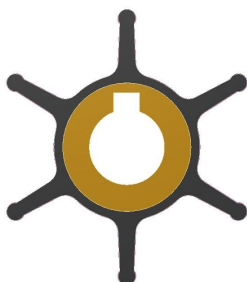
Cod. 5357: De 40 - H 12.6 - Di 10.8, Neoprene, Ins. 3
