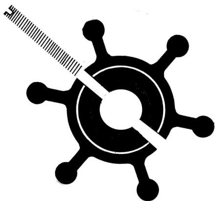
Cod. 3398: De 51 - H 22 - Di 8, Neoprene, Ins. 1 Cod. 3399: De 51 - H 22 - Di 8, Nitrile, Ins. 1
