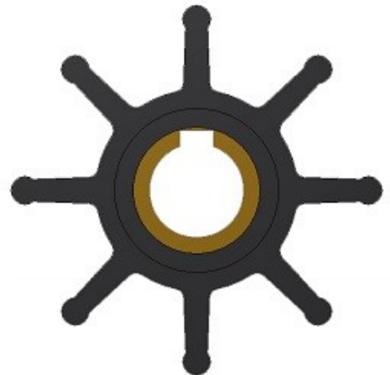
Cod. 6508: De 80 - H 75 - Di 20, Neoprene, Ins. 3
