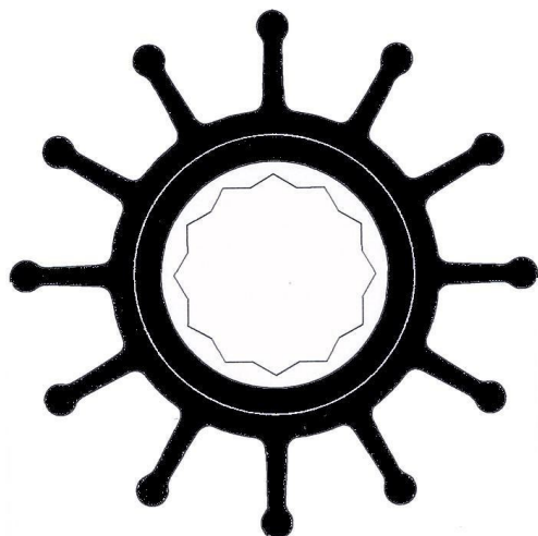
Cod. 4205: De 65 - H 80 - Di 25.48, Neoprene, Ins. 4
