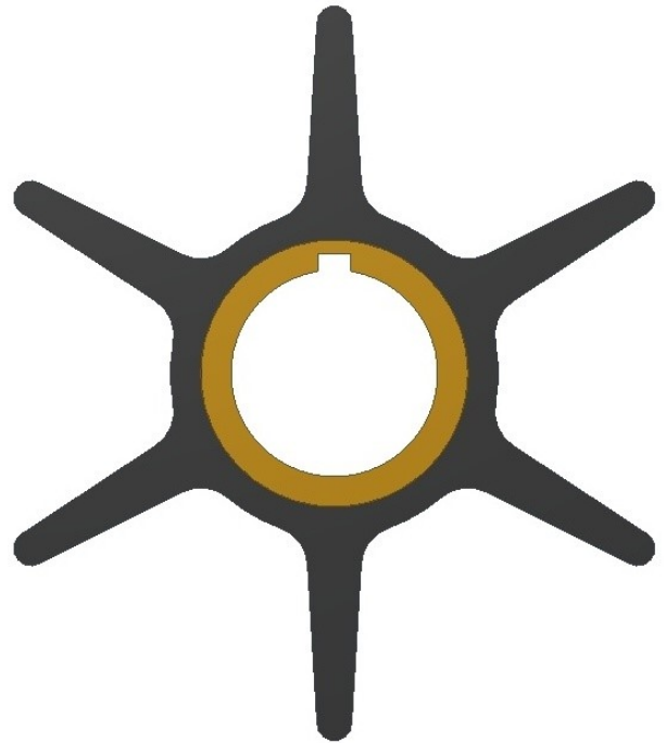
Cod. 6003: De 90 - H 31.2 - Di 26, Neoprene, Ins. 3
