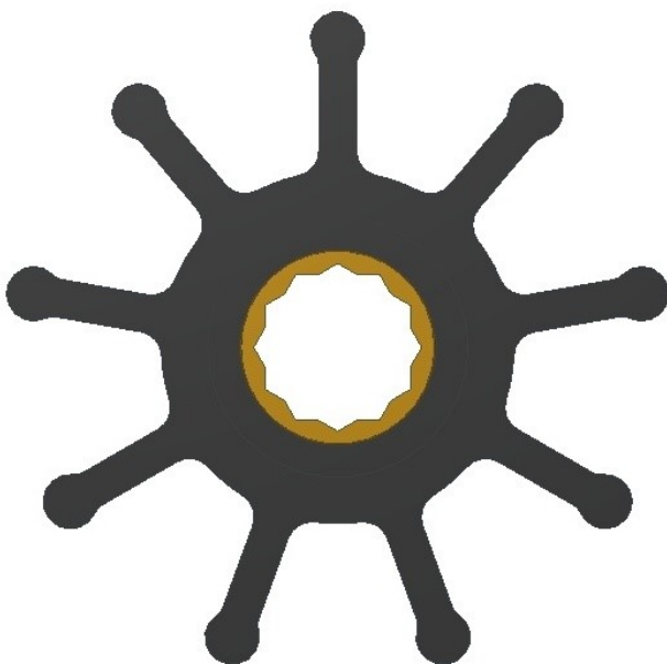
Cod. 5886: De 80 - H 75 - Di 20, Neoprene, Ins. 4 Cod. 6088: De 80 - H 54 - Di 20, Neoprene, Ins. 4
